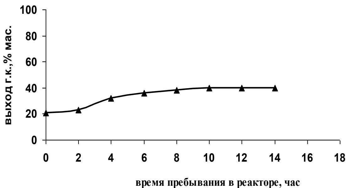
Рис. 2. Зависимость выхода гуминовых кислот от времени пребывания угля в реакторе (в присутствии острого водяного пара)
