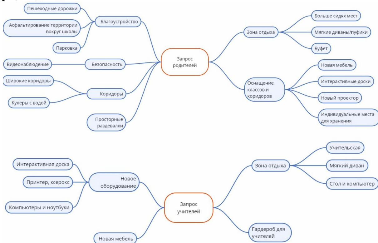
Рис. 3. Систематизация запросов
