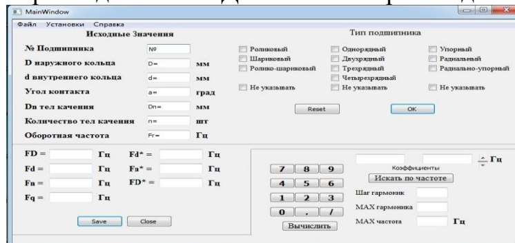
Рисунок 3. Интерфейс программы.
