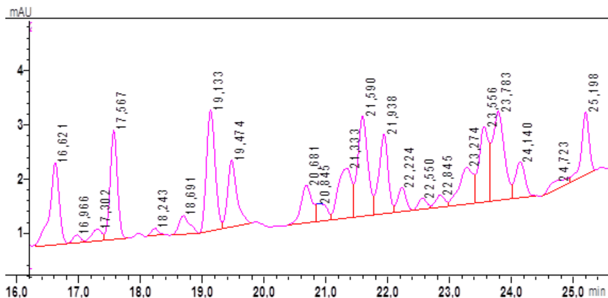
Рис. 1. Хроматограмма образца талого снега
