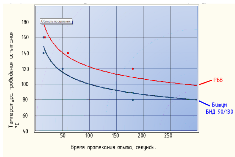
Рис. 1. Зависимость условной вязкости битума БНД 90/130 и резинобитумного вяжущего (РБВ) от температуры
