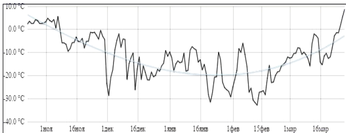
Рис. 1. Изменение температуры почвы в осенне-зимний-весенний период за 2006-2007, 2007-2008 и 2008-2009 года соответственно
