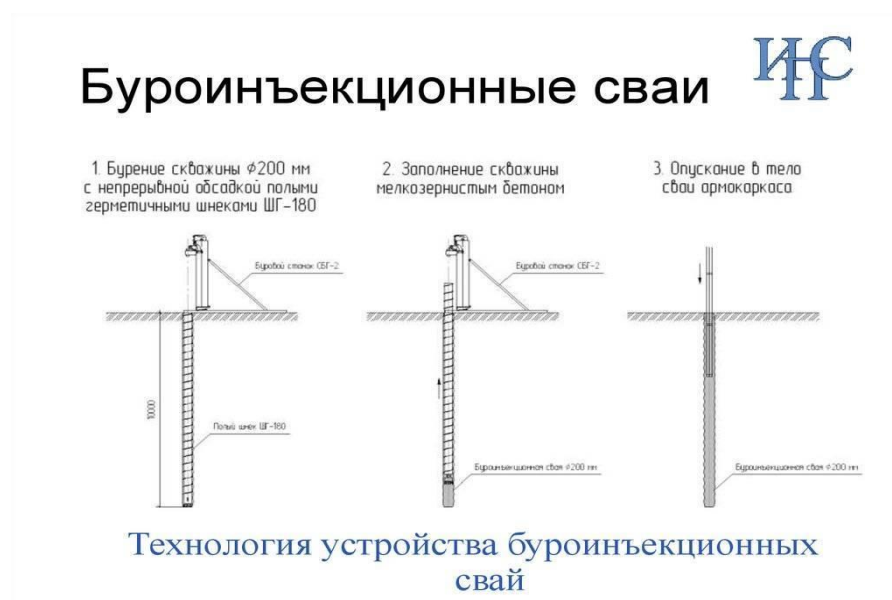
Рисунок 1. Буроинъекционно-компенсационные сваи
