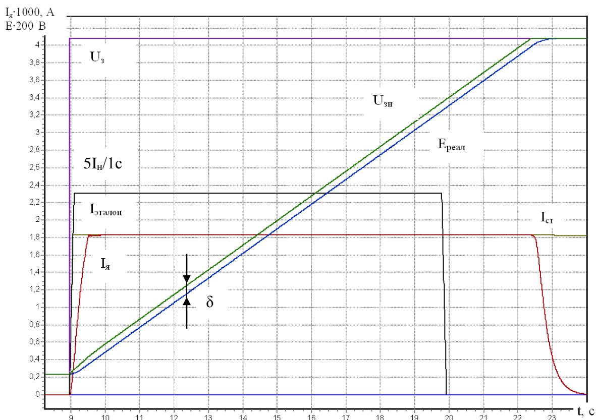
Рисунок 3 – Переходный процесс в системе с токоограничением
