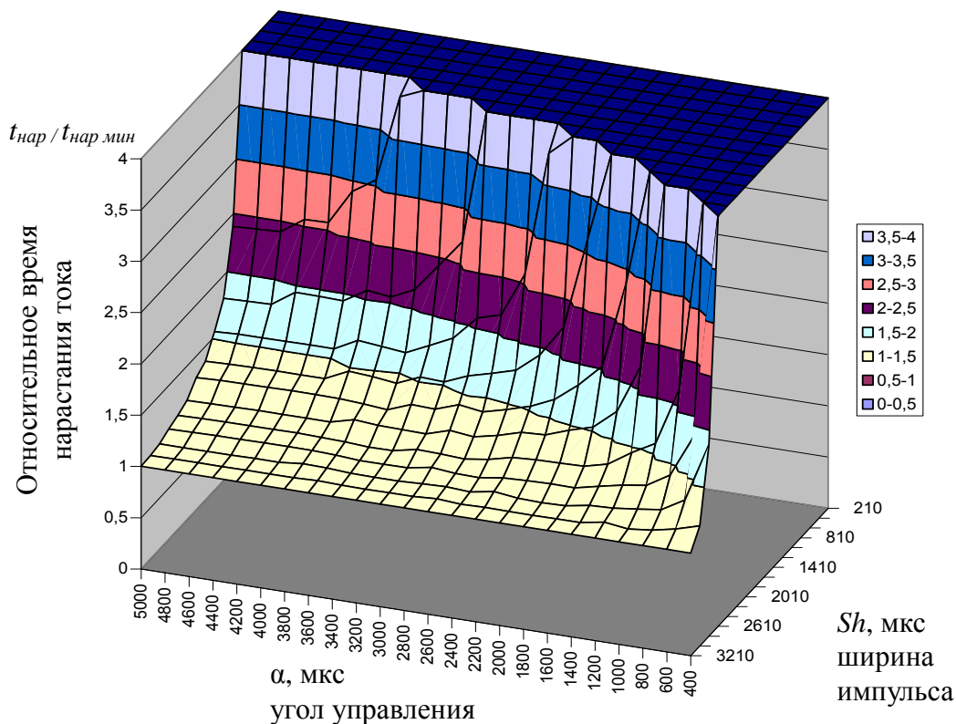
Рисунок 1 – График зависимости относительного затягивания времени реверса в функции ширины импульса Sh и угла управления \alpha
