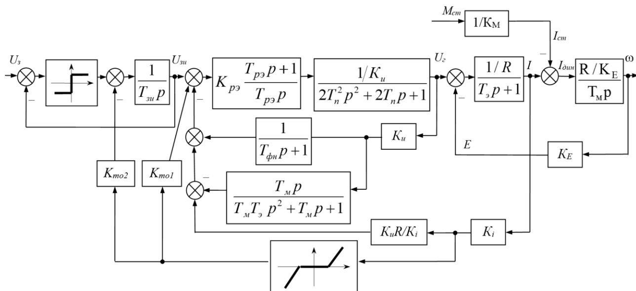
Рисунок 2 – Структура системы автоматического регулирования скорости с токоограничением
