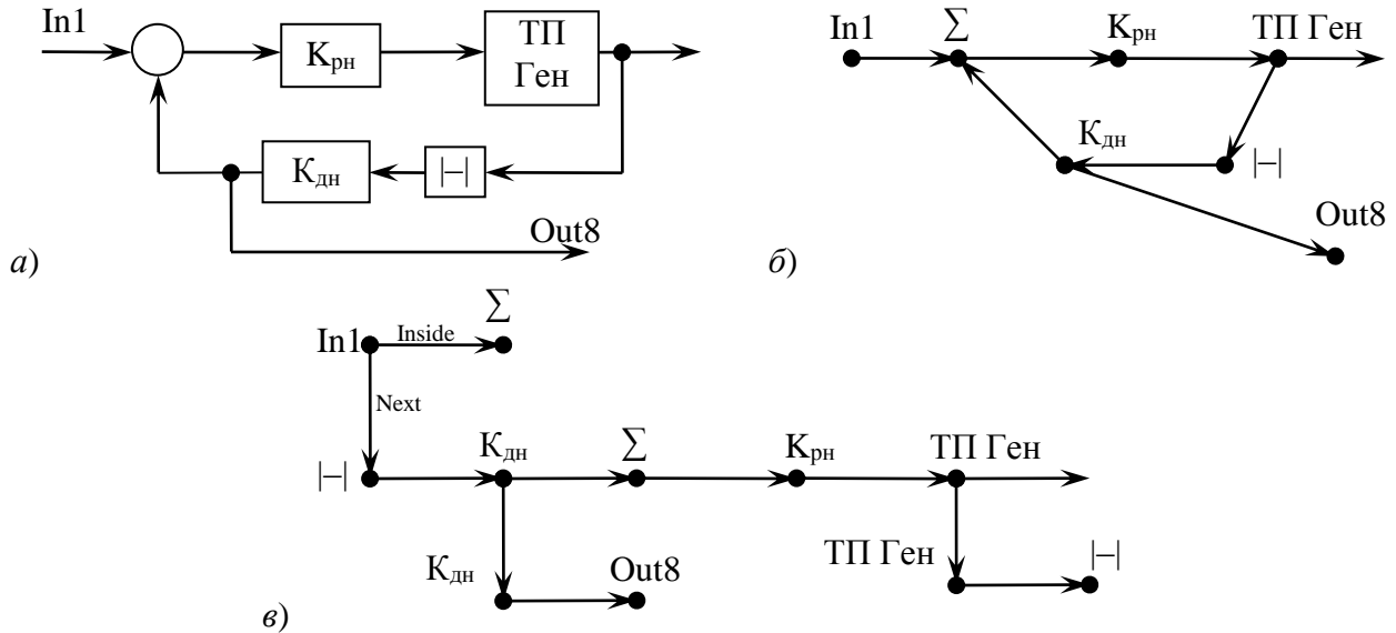
Рисунок 4 – Модель контура напряжения (а), граф модели (б) и дерево модели (в)
