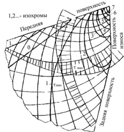
Рис. 2 Изохромы
