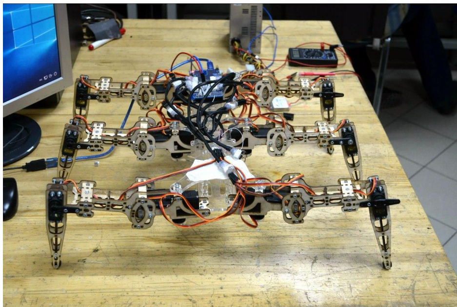
Рисунок 2. Конструкция робота на текущий момент
