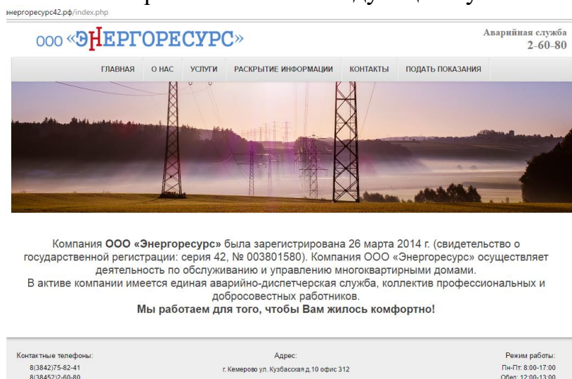
Рис. 1. Главная страница
