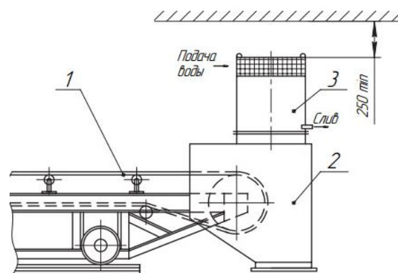
Рис. 2. Схема установки аппарата ПР-ТАЙРА-5000 1 – конвейер; 2 – укрытие места разгрузки конвейера; 3 – пылеулавливающий аппарат
